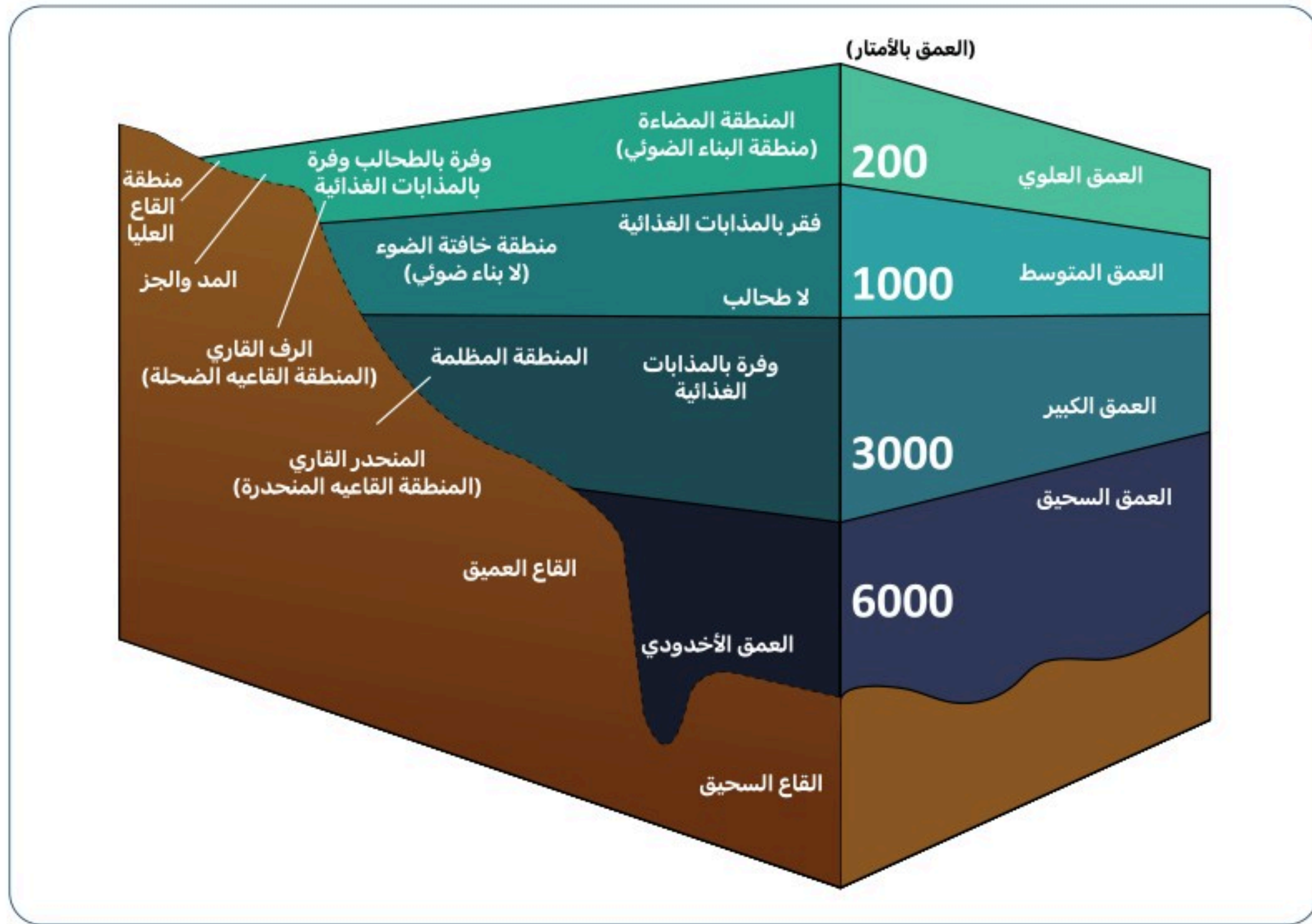
شكل 18-8 أقسام النظم البيئية البحرية.
