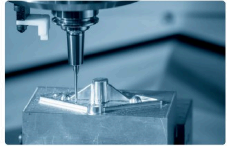
شكل 2.13: عملية التصنيع من خلال الإزالة
