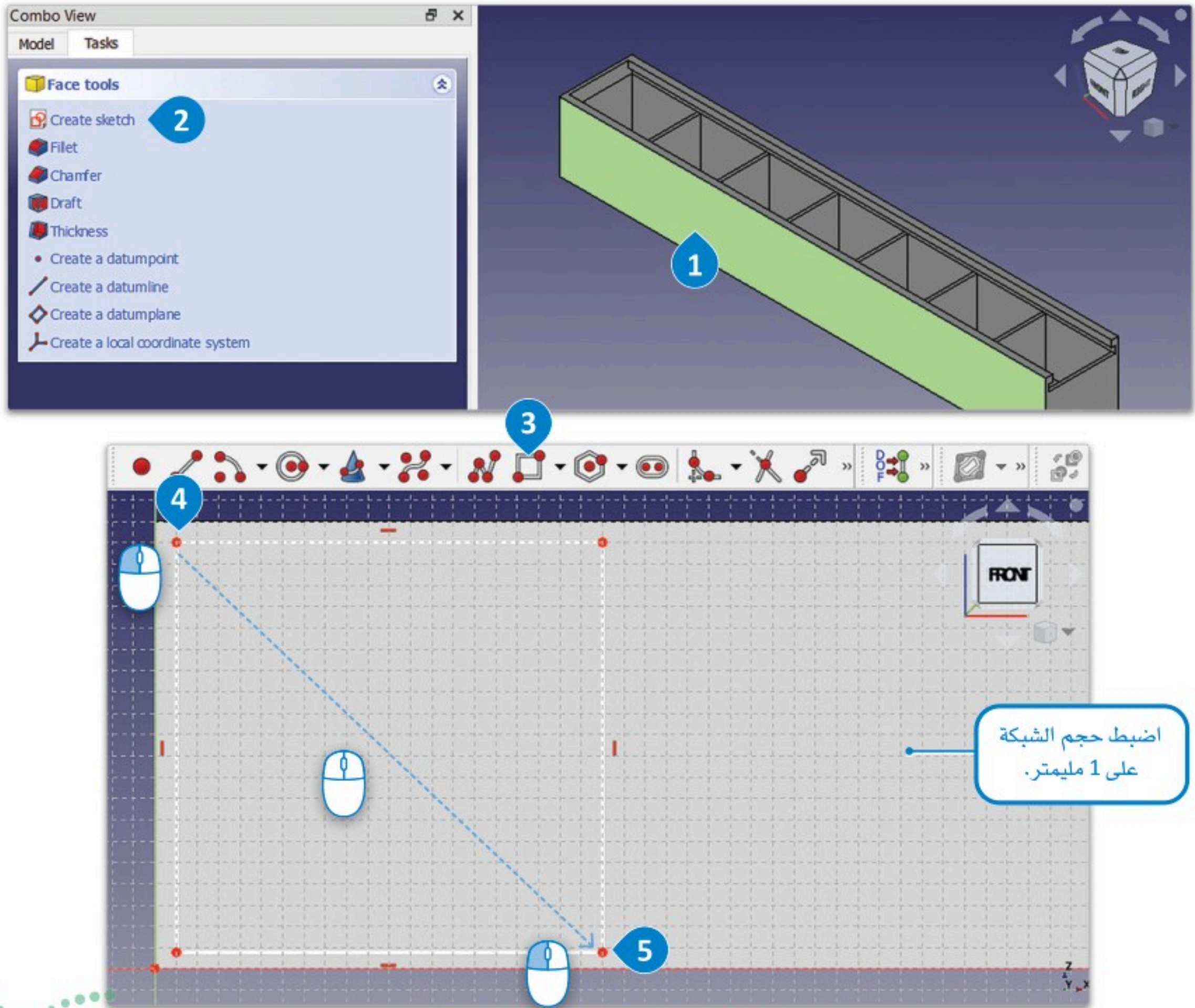
شكل 3.51: إنشاء رسم تخطيطي على سطح الصندوق
