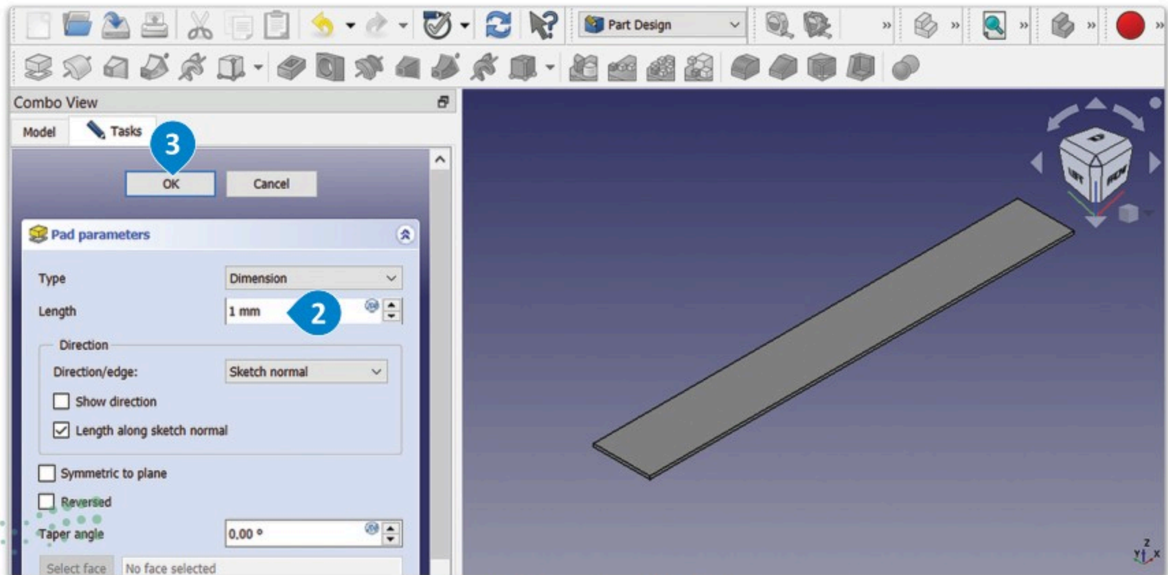
شكل 3.61: إنشاء غطاء صندوق أقراص الدواء
