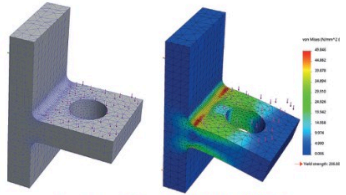
شكل 2.9: تحليل العناصر المحدودة ناتج عن نموذج صلب
