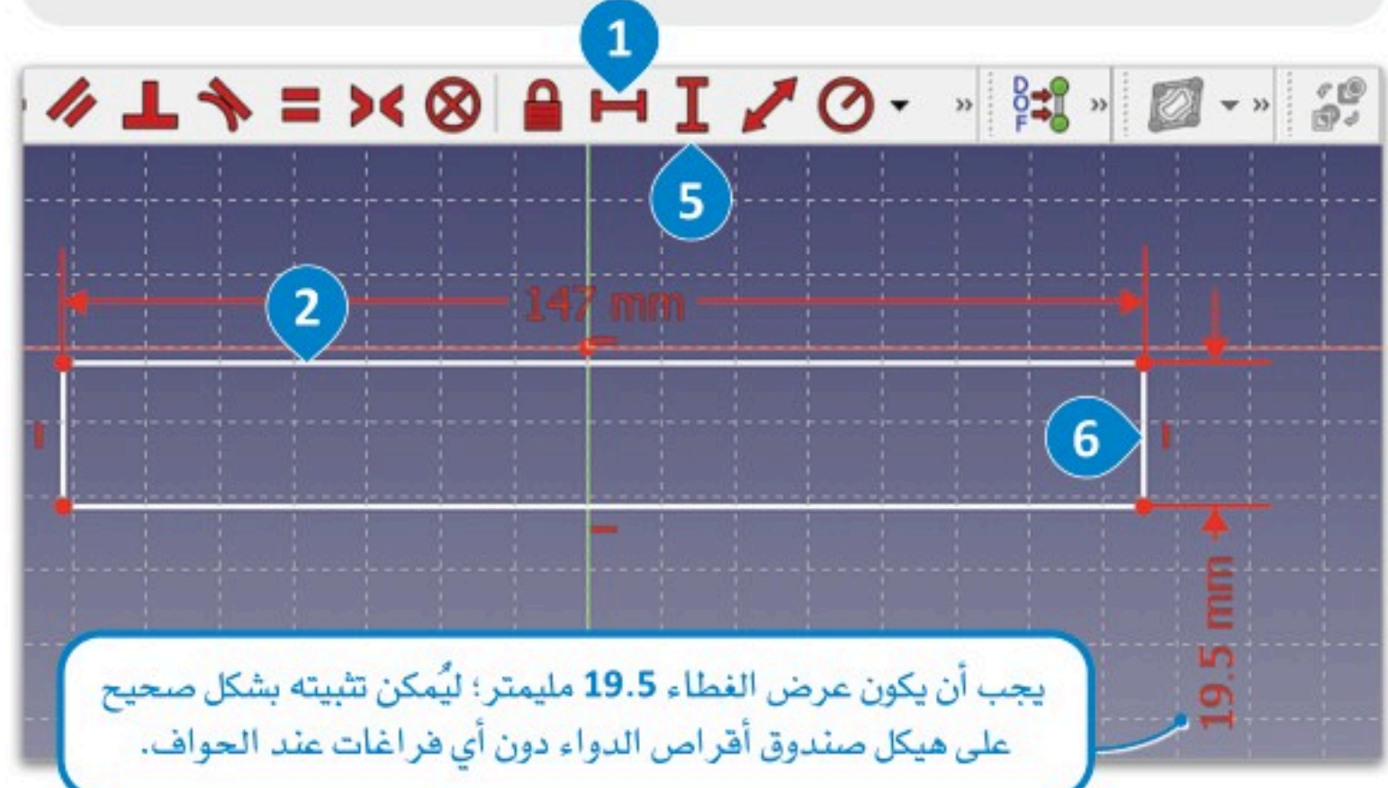
شكل 3.60: تقييد المسافة الأفقية والرأسية
