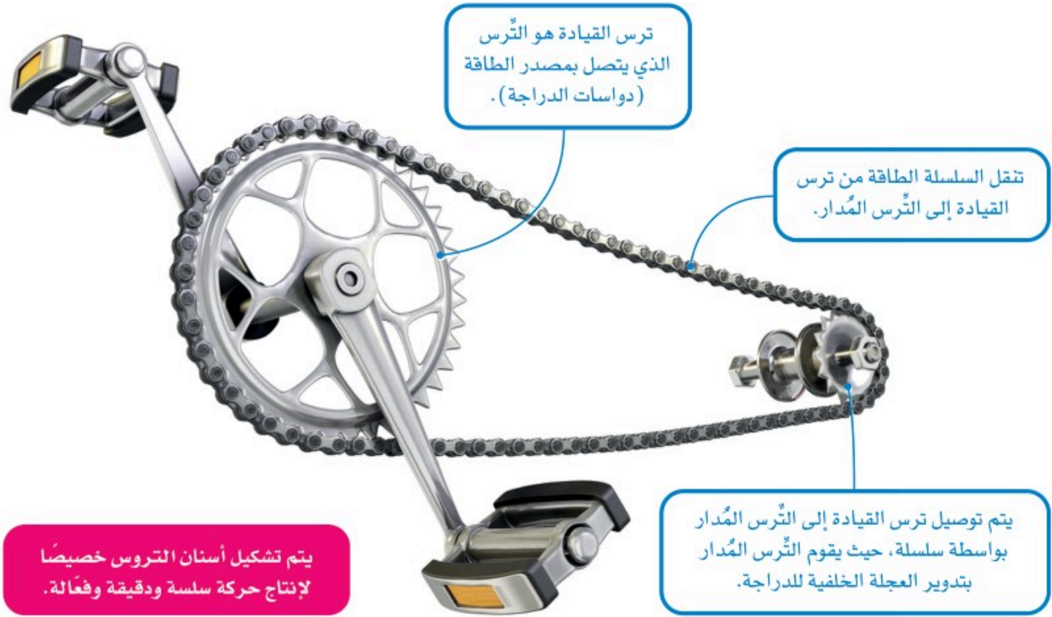
شكل 2.41: آلية الحركة في الدراجة
