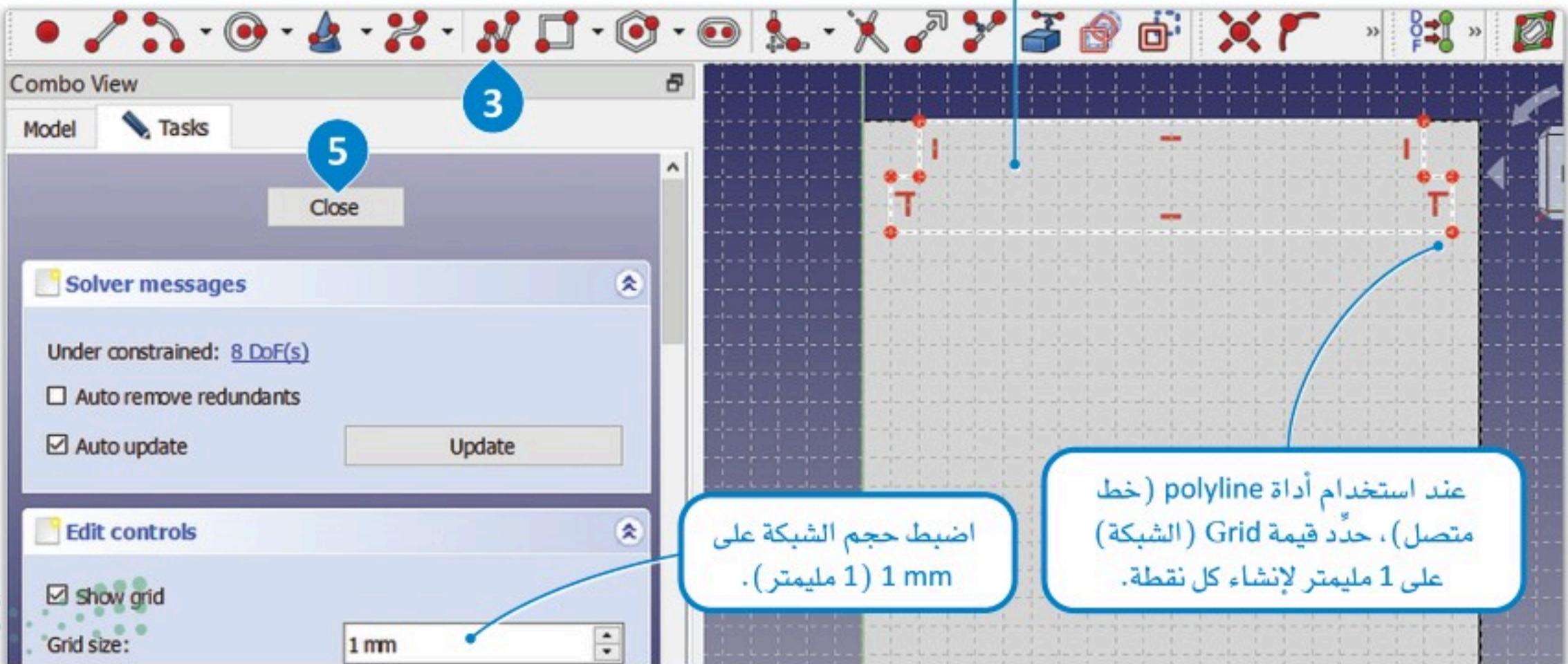
شكل 3.47: إنشاء رسم تخطيطي على السطح العلوي
