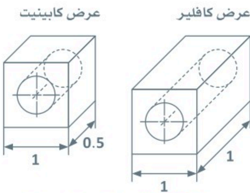
شكل 2.15: مثالان على الرسم الهندسي المائل
