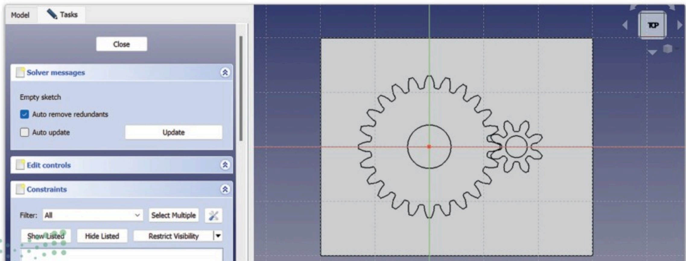
شكل 2.62: إنشاء رسم تخطيطي على السطح العلوي للقاعدة
