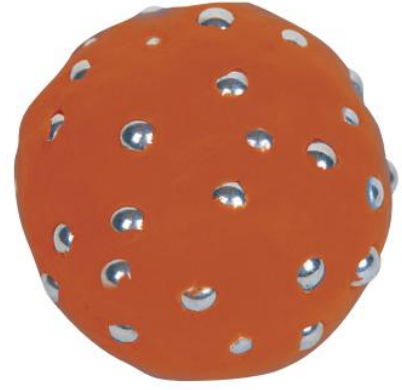
الشكل ٨ نموذج كرة الصلصال التي تحوي كرات صغيرة منتشرة فيها، هو طريقة أخرى لتصوير الذرة؛ حيث تحوي كرة الصلصال كل الشحنات الموجبة، والكرات الصغيرة تُمثِّل الشحنات السالبة. فسّر لماذا ضمَّن طومسون الجسيمات الموجبة في نموذجهِ للذرة؟
