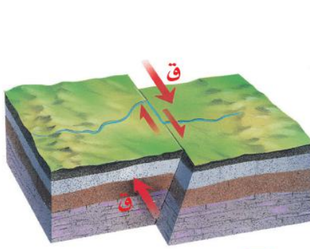
ج ينتج الصدع الجانبي (الانزلاقي) عندما تتعرض الصخور لإجهادات قص (تؤثر فيها بصورة جانبية).
