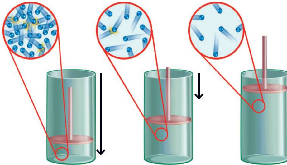
الشكل ١٩ بتقصان حجم الغاز المحصور يزداد الضغط. يقل الحيز الذي تشغله جسيمات الغاز بحركة المكبس إلى أسفل فيزداد عدد تصادماتها، لذا يزداد الضغط.
