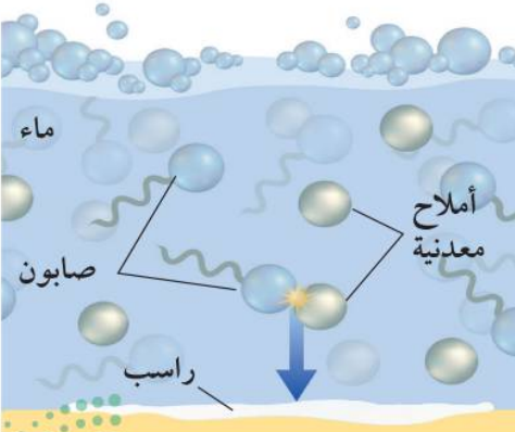
الشكل ٣ تتفاعل الأملاح مع الصابون فتشكل راسباً.
