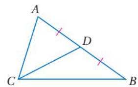
\overline{CD} قطعة متوسطة في \triangle ABC .
