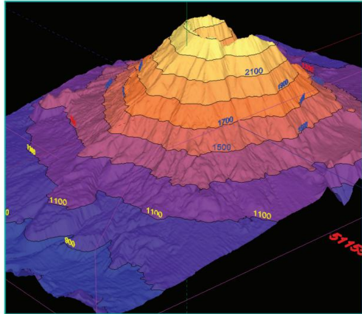
خطوط الكُنْتُور
