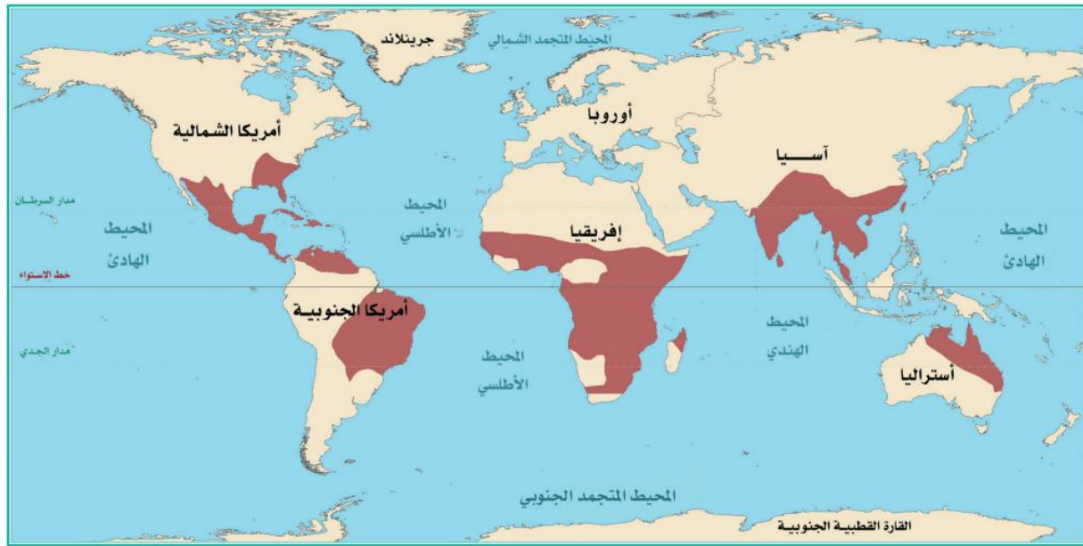
الإقليم المداري
