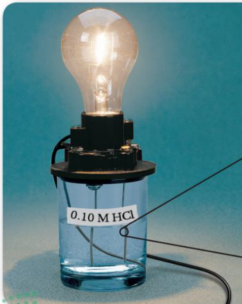
الشكل 2-11 يتوهج المصباح بقوة عندما يوضع القطبان في محلول حمض الهيدروكلوريك بتركيز 0.10 M؛ لأن جميع HCl تتحلل إلى أيونات هيدروجين وأيونات كلوريد.
