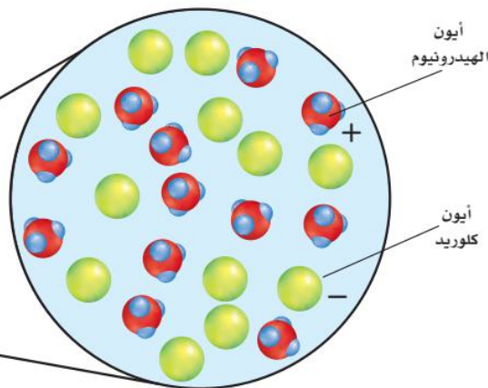
الشكل 2-11 يتوهج المصباح بقوة عندما يوضع القطبان في محلول حمض الهيدروكلوريك بتركيز 0.10 M؛ لأن جميع HCl تتحلل إلى أيونات هيدروجين وأيونات كلوريد.
