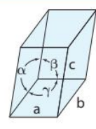
ميكروكلاين
