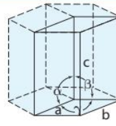
تورمالين
