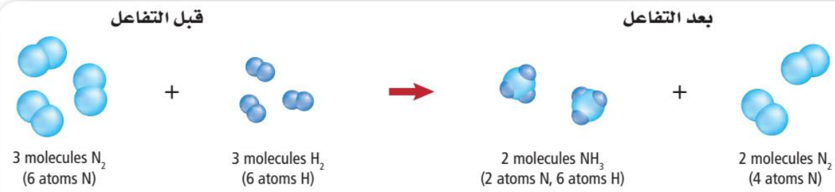
الشكل 5-12 إذا أمعنت النظر في الذرات الموجودة قبل التفاعل وبعده فستجد أن بعض جزيئات النيتروجين لم تتغير. وتسمى هذه الجزيئات المادة الفائضة.
