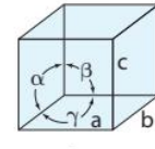
هالايت
