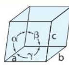
زمرد
