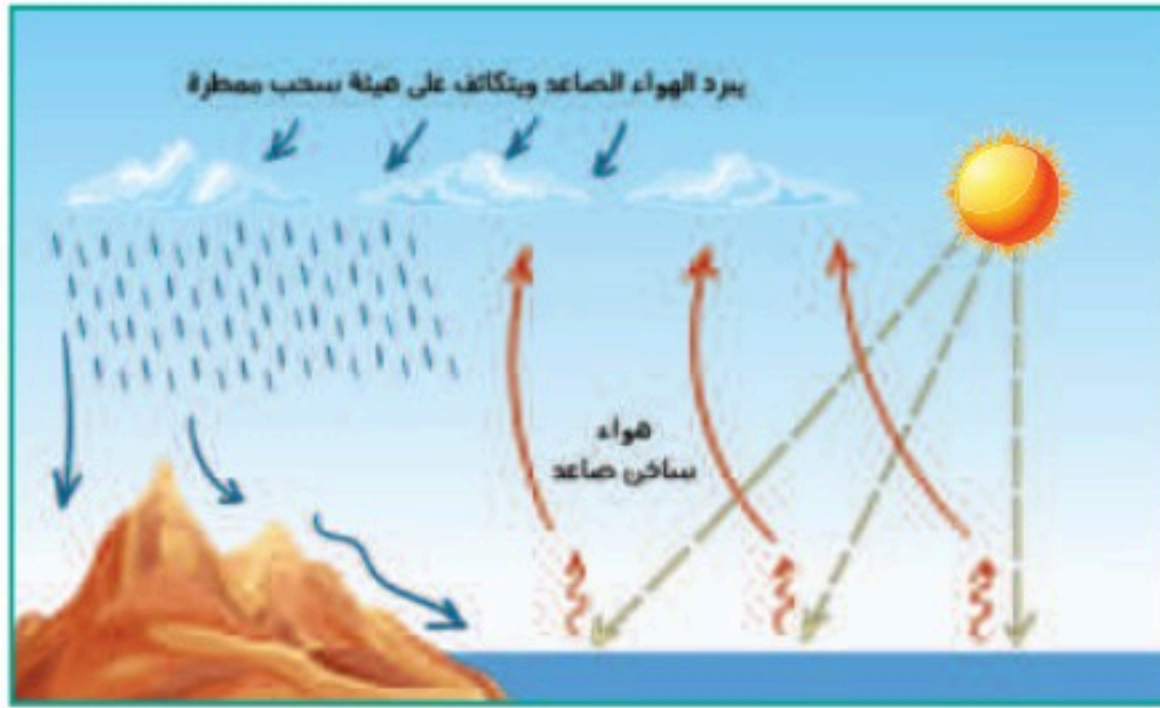
المطر التصاعدي
