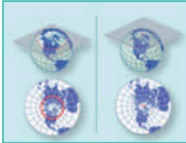
المسقط المستوي
