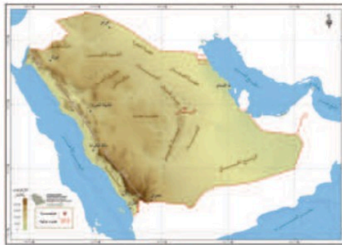
خريطة تضاريسية
