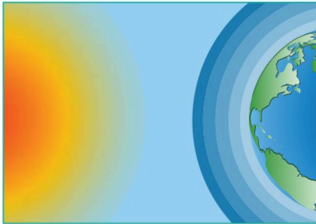
الغلاف الجوي
