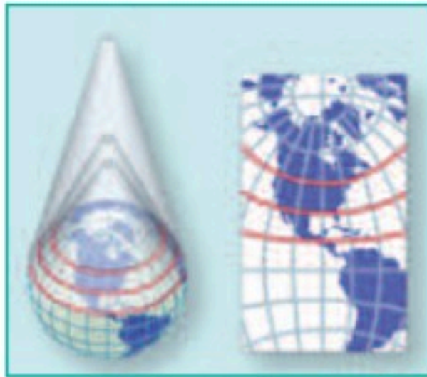
المسقط المخروطي
