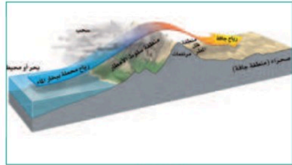
المطر التضاريسي
