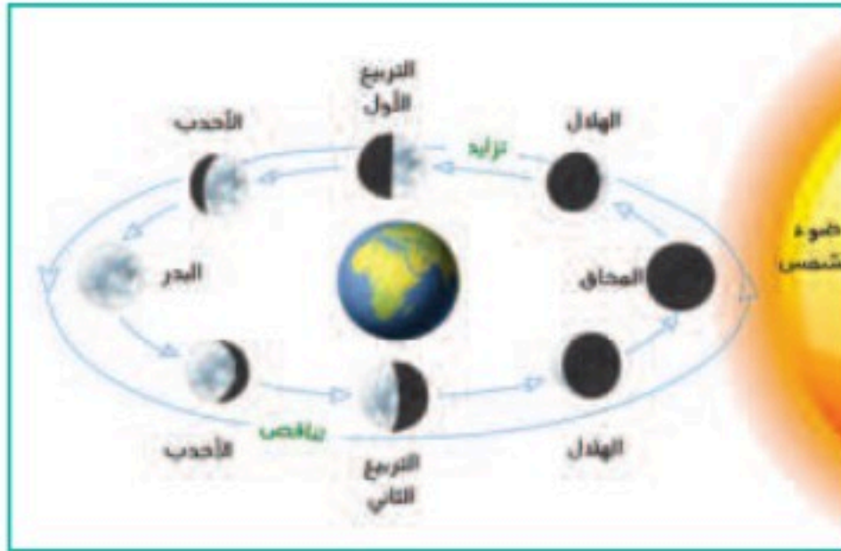
أوجه القمر
