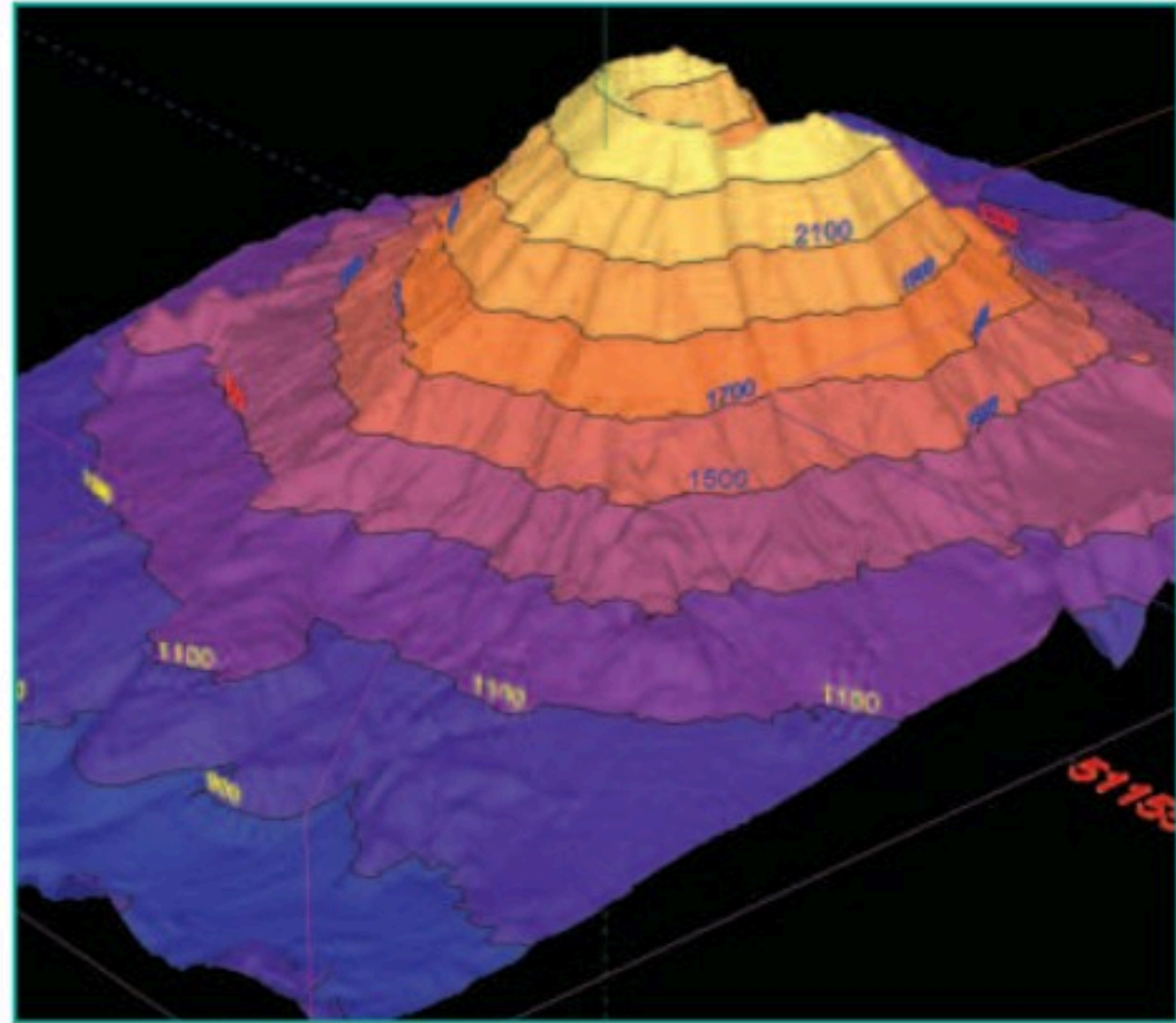
خطوط الكُنْتُور
