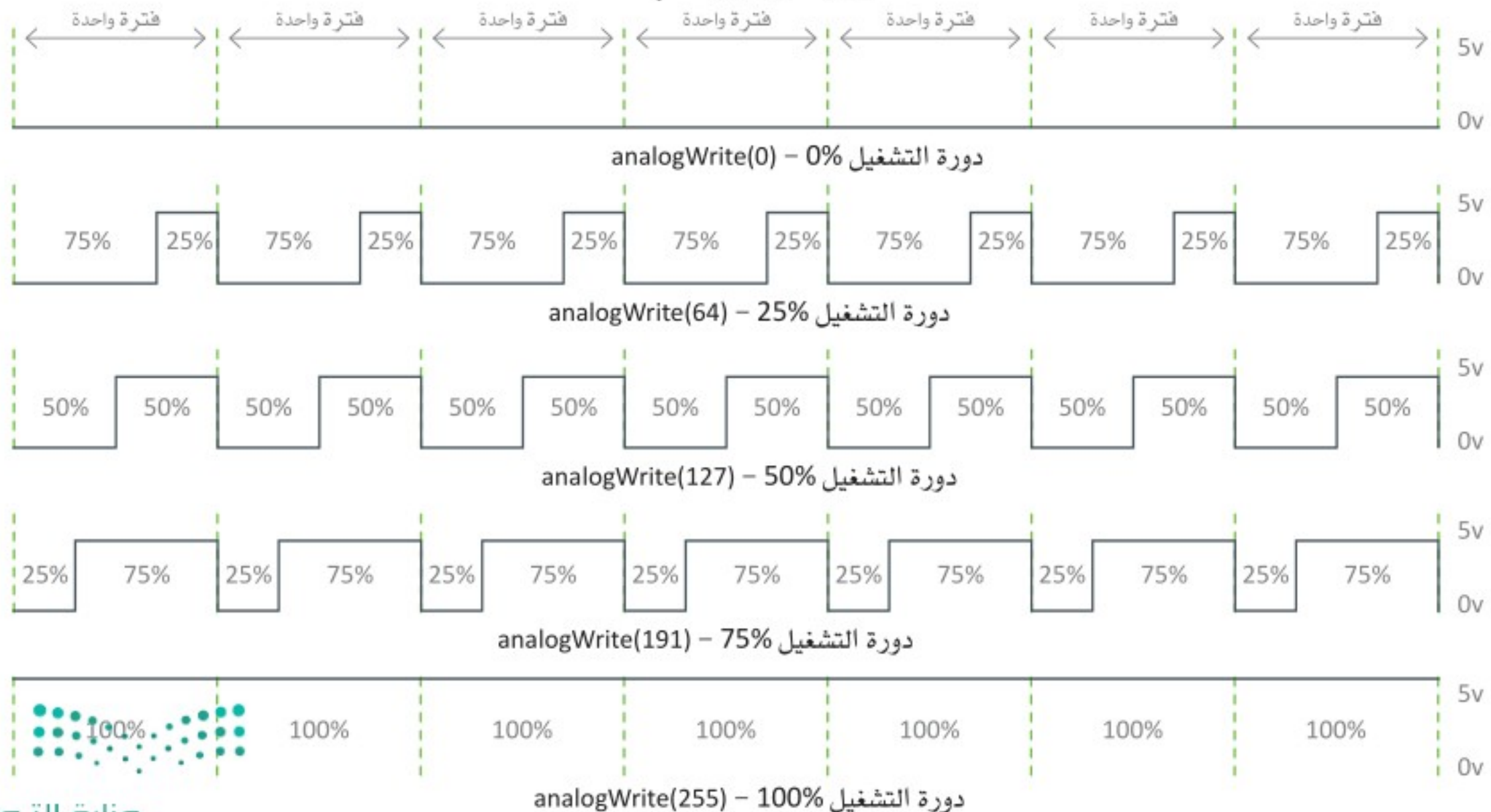
شكل 4.6: تضمين عرض النبضة
