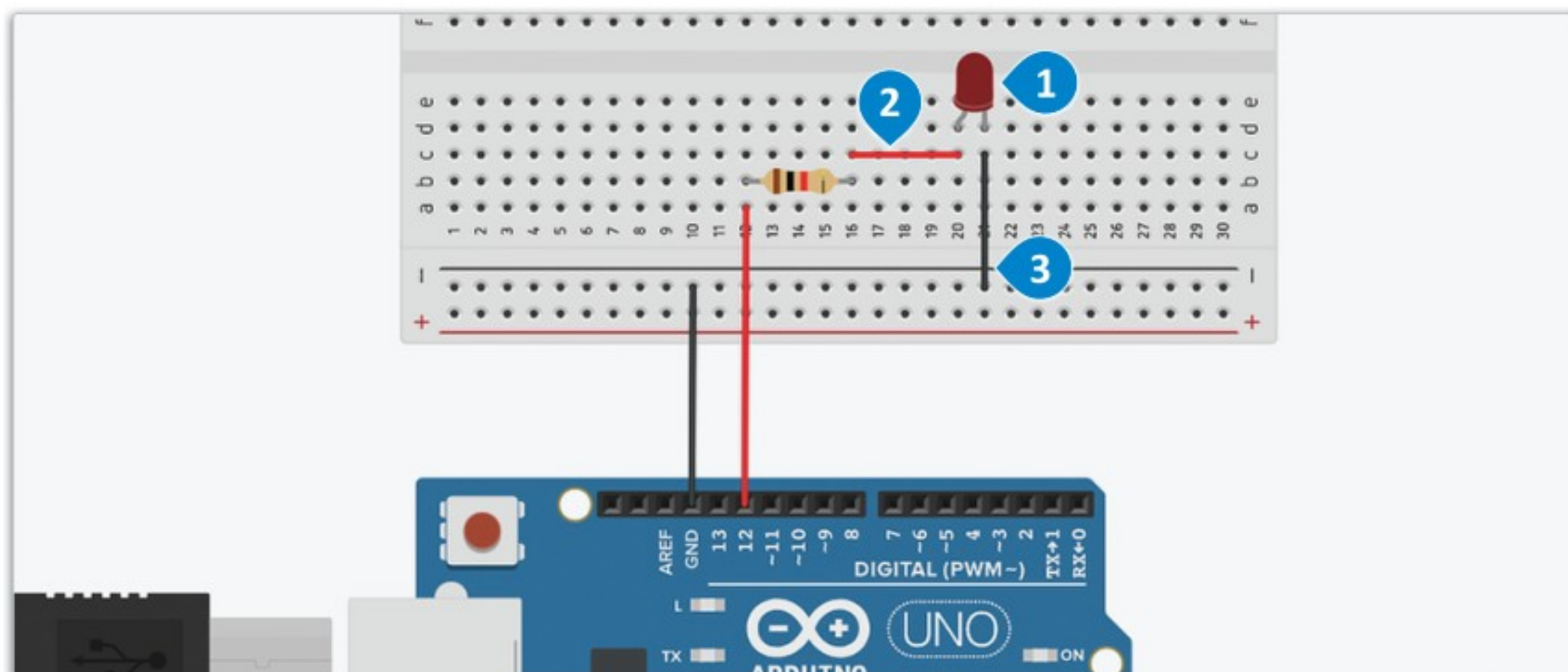
شكل 4.11: توصيل الدايود المشع للضوء الخارجي
