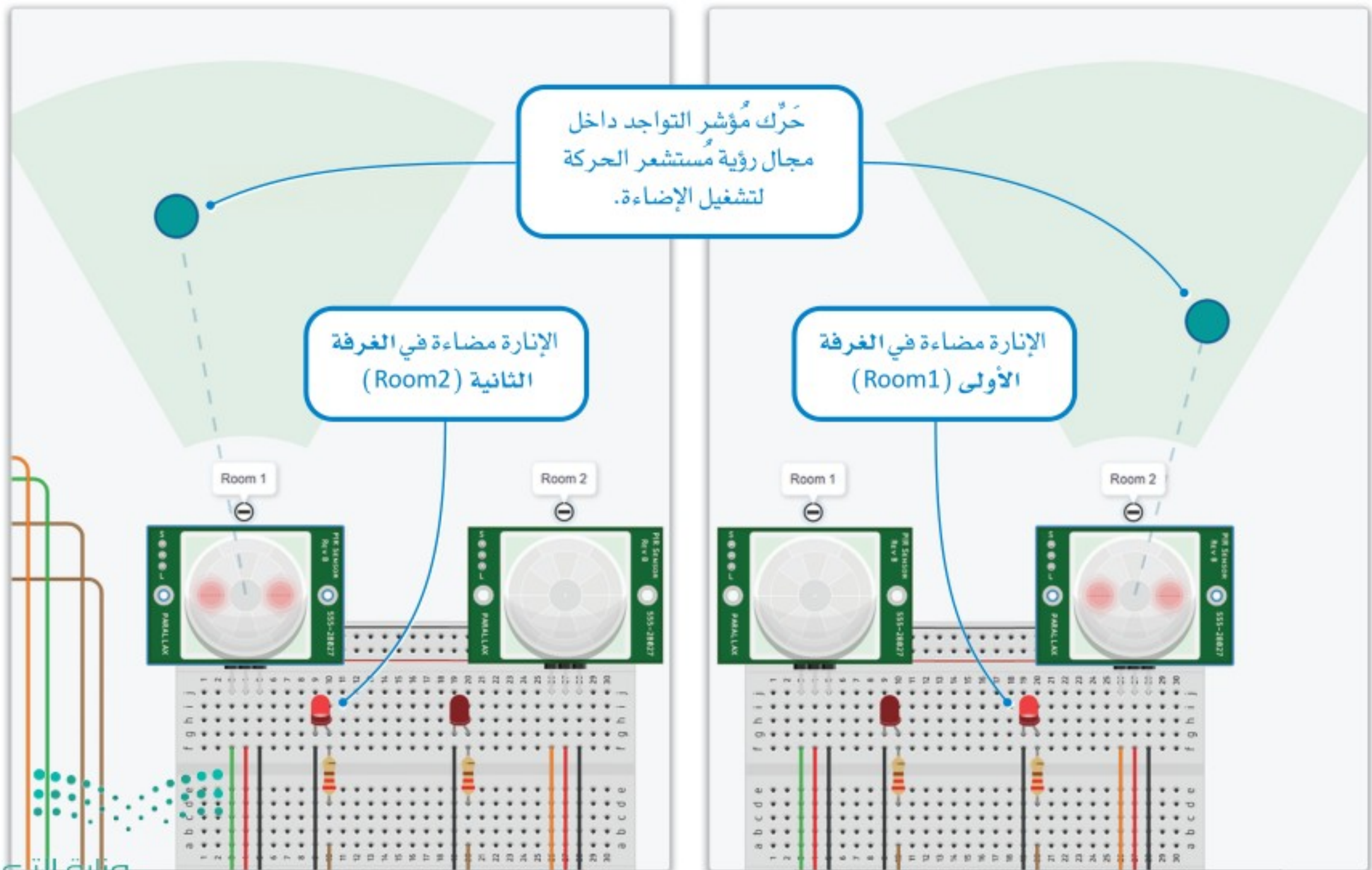
شكل 3.18: محاكاة البرنامج
