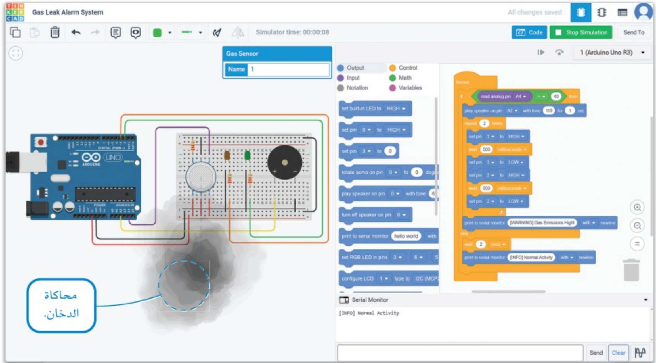
شكل 3.41: تنفيذ البرنامج
